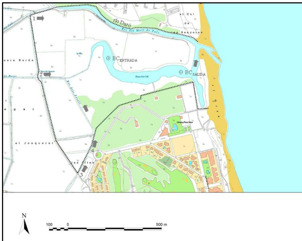
Figura 2. Mapa detallado de la laguna “les Basses d’en Coll”. Se indica el flujo preferencial del agua dulce a través del ecosistema, los puntos de entrada de agua dulce muestreados (del 1 al 4) y los puntos muestreados en el interior de la laguna, BC_{ENTRADA} y BC_{SALIDA} . En línea discontinua se delimita el perímetro global del Espacio Natural Basses d’en Coll .
